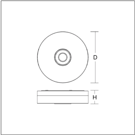
Plafond- en wandarmaturen 4051859255017 D 300, H 95 Plafondmontage (opbouw), Wandmontage rvs geborsteld
