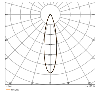
FL PFM 150W 4000K SYM R30 BK
