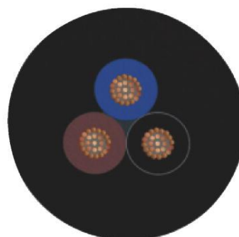
Cable
