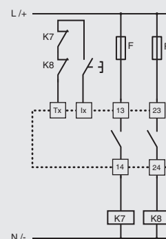
Circuit de rétroaction pour les contacteurs externes avec démarrage manuel ou contrôlé
