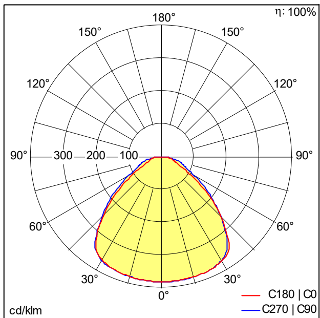
TE_ZOE_VARIO_200_2000_840_DALI.ltd
