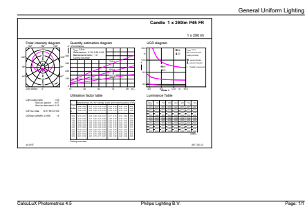
CorePro LEDlustre 25W E14 840 FR P45
