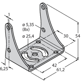
U-vormige bevestigingsklem voor montage op de grond (bevat grondplaat SMBIVUB)
