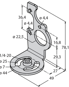
bevestigingsklem monteerbaar linkerzijde
