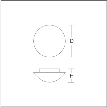
Plafond- en wandarmaturen 4051859030003 D 370, H 118 Plafondmontage (opbouw), Wandmontage zuiver wit (RAL 9010)
