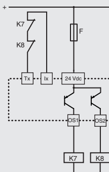
Zpěnovazební obvod pro externí stykače s automatickým startem
