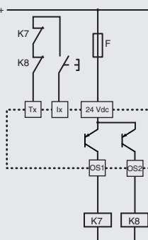
Zpěnovazební obvod pro externí stykače s ručním nebo monitorovaným startem
