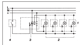
1. Nulla vezető nélküli világítótések
