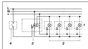
1. Lamp zonder aanwezige nuldraad
