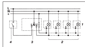
2. Nulla-vezetékkel rendelkező világítótések
