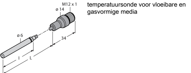
TP-504A-TRI3/4-H1141-L035 9910429
