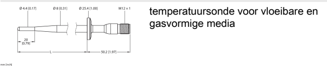
TP-504A-TRI3/4-H1141-L035 9910429
