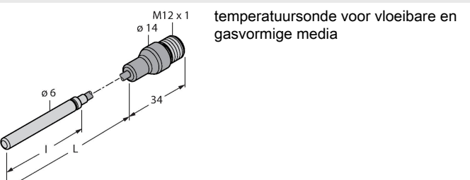
TP-306A-CF-H1141-L5000 9910481
