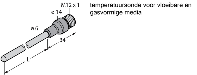
TP-306A-CF-H1141-L2000 9910480
