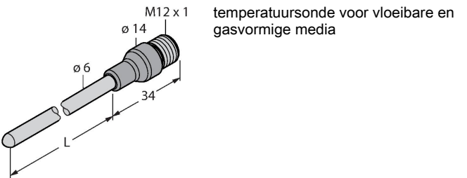
TP-206A-CF-H1141-L300 9910478
