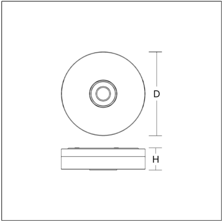
Plafond- en wandarmaturen 4051859254973 D 300, H 95 Plafondmontage (opbouw), Wandmontage rvs geborsteld
