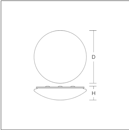
Plafond- en wandarmaturen 4051859431275 D 460, H 120 Plafondmontage (opbouw), Wandmontage wit
