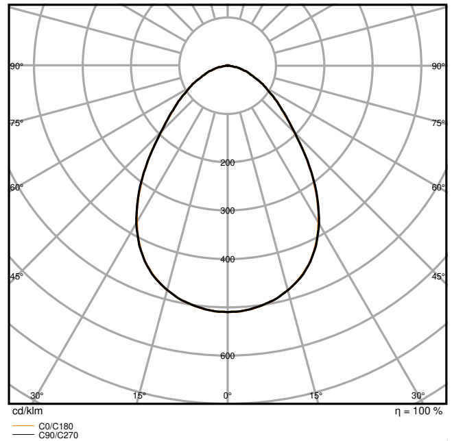
PL PROT 600 P 36W 840 U19 DALIVR 5040lm
