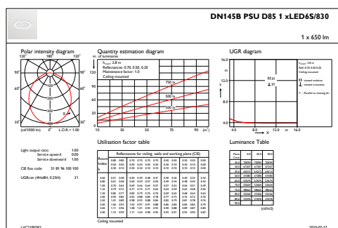
IFGU1_DN145BPSUD851xLED6S830
