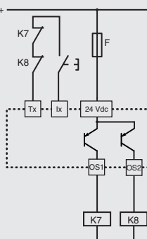
Zpětnovazební obvod pro externí stykače s ručním nebo monitorovaným startem
