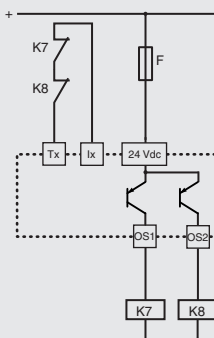
Zpětnovazební obvod pro externí stykače s automatickým startem
