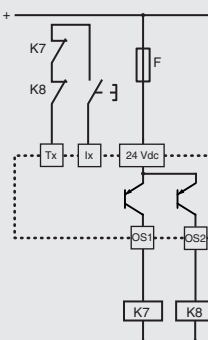
Circuit de rétroaction pour les contacteurs externes avec démarrage manuel ou contrôlé
