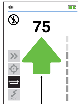
Leitungsschutzschalter/Sicherung gefunden
