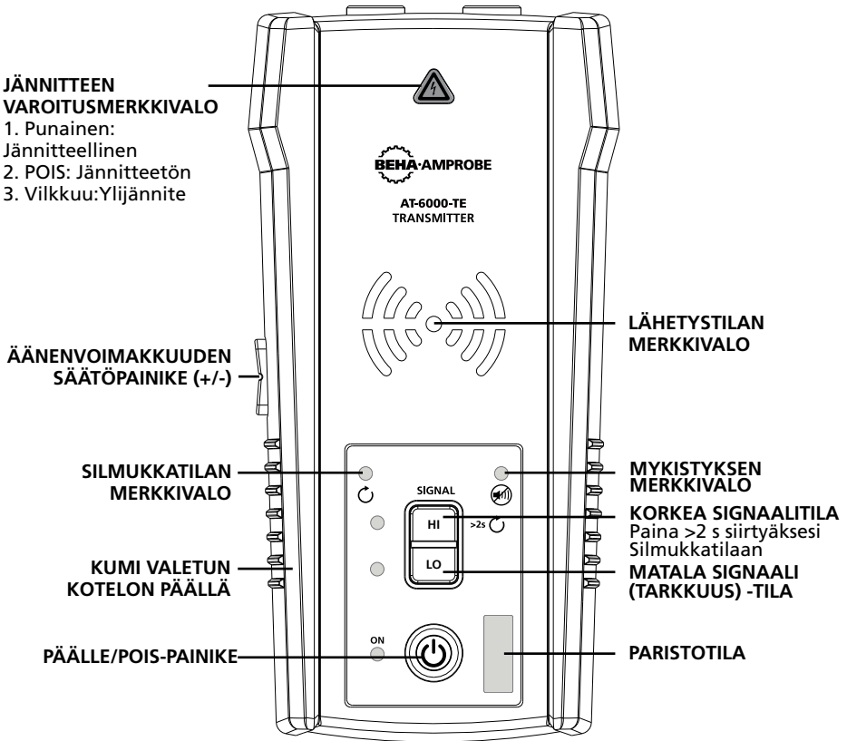
Kuva 2.2e: AT-6000-TE-lähettimen yleiskatsaus
