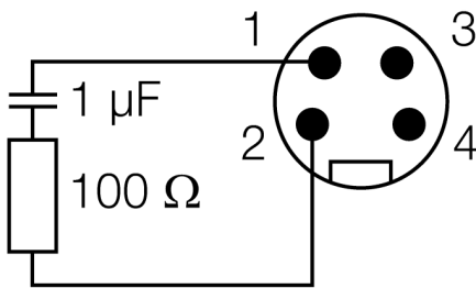
Aansluitschema
