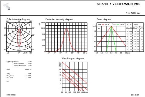
IFAS1_ST770T1xLED27SCHMB
