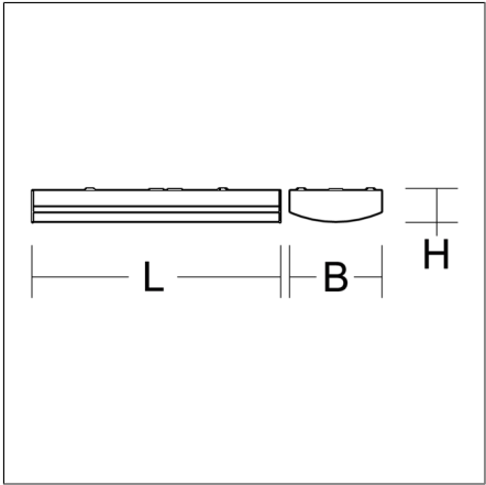
Plafond- en wandarmaturen 4051859765783 L 600, B 160, H 58 Plafondmontage (opbouw), Wandmontage verkeer wit, mat (RAL 9016)
