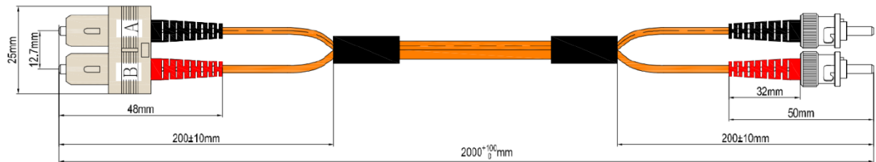
Maßzeichnung (Beispiel 29021102)
