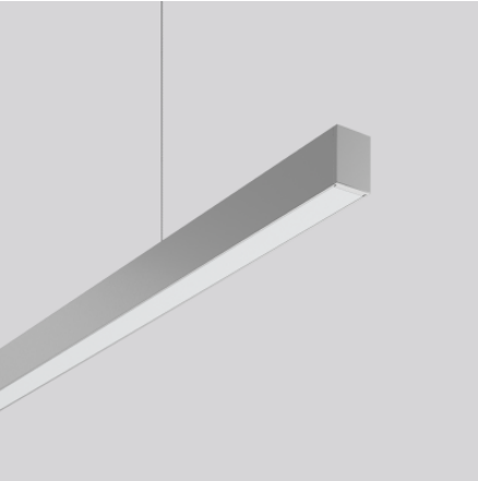
Pendant luminaires 4051859999867 L 1512, B 28, H 38 pendant silver, matt (approx. RAL 9006)
