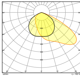
FL PFM 150W 3000K ASYM 55x110 BK
