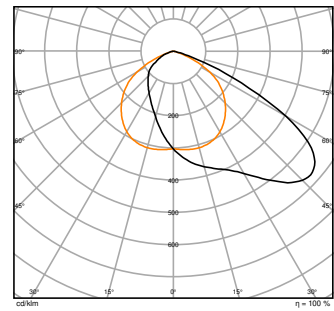
FL PFM 150W 3000K ASYM 55X110 BK
