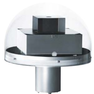
Tageslichtmesskopf mit Busanschluss zur Erfassung des Himmelzustandes mit 8 abgeglichene Fotozellen
