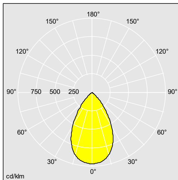
TLG_CHAL3_150_2000-830_EHF_RSB.ltd
