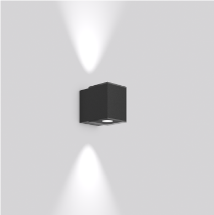
Wandleuchten 4051859753612 L 100, B 154, H 127 Wandanbau anthrazit metallic (DB703)
