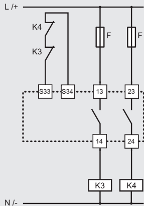
Rückführkreis für externe Schütze mit automatischem Start
