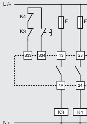
Rückführkreis für externe Schütze mit manuellem oder überwachtem Start
