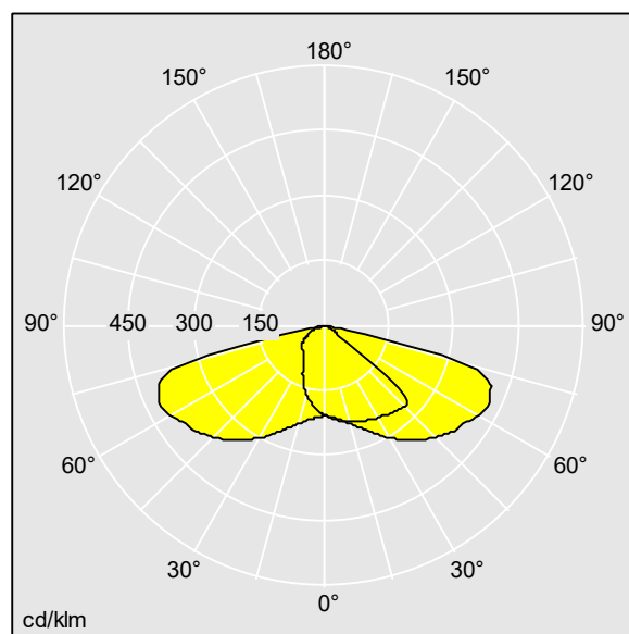
TL_IS24L70NR730.idt
