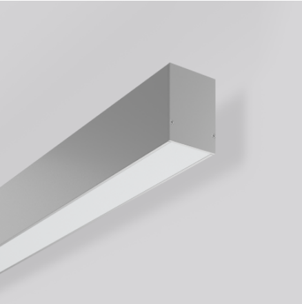
Luminarias de pared 4068754009607 L 1687, B 67, H 75 Montaje en superficie de la pared aluminio, mate (aprox. RAL 9006)
