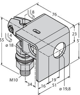
montagebeugel, materiaal VA 1.4401, voor 18 mm schroefdraad, schroefdraad M10 x 1,5
