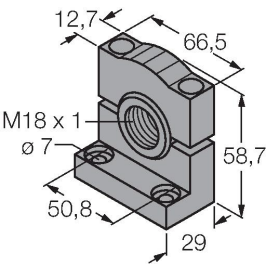
montagebeugel, PBT-zwart, voor sensoren voor 18mm schroefdraad
