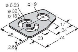
montageplaat, roestvast staal, voor sensoren met 18mm schroefdraad
