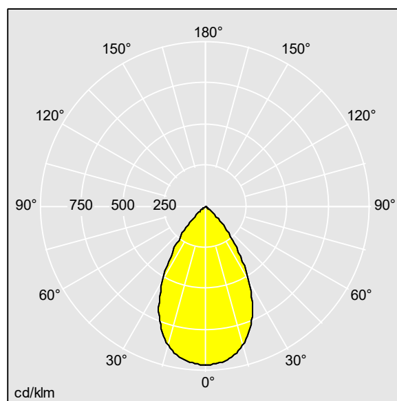
TLG_CHAL3_150_2000-830_HFIX_RSB.ltd
