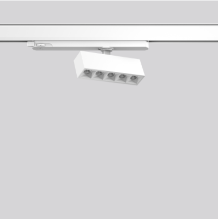
Proyectores 4051859744368 L 145, B 35, H 80 Carril de corriente en el techo, Carril de corriente en la pared blanco tráfico mate (RAL 9016)
