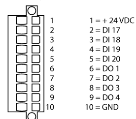
Pinbezetting CN7
