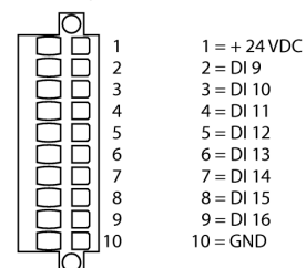
Pinbezetting CN6
