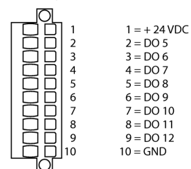
Pinbezetting CN8
