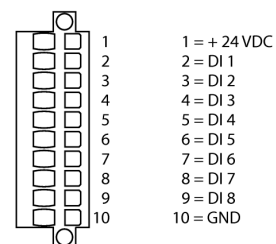
Pinbezetting CN5
