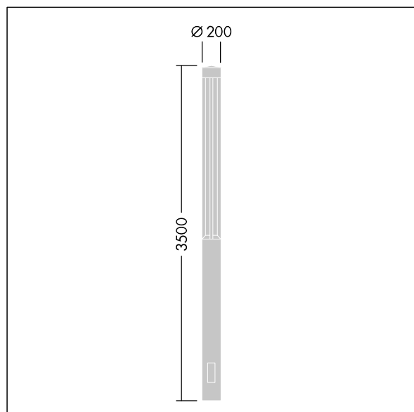
TLG_CESA_M_STRUT_H3500.wmf
