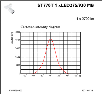
IFCC1_ST770T1xLED27S930MB
