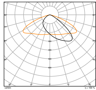
FL PFM 150W 4000K ASYM 45X140 BK
