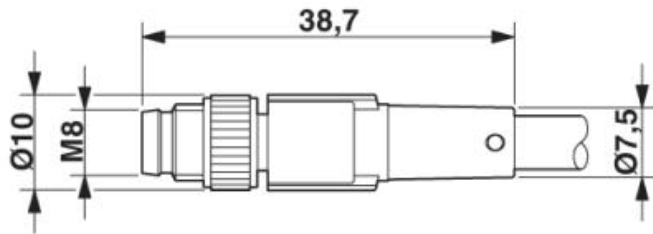
Maßzeichnung, M8 Stecker
