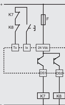
Zpětnovazební obvod pro ruční nebo monitorovaný startem
