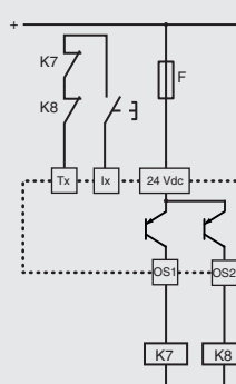
Circuito de retorno para contactores externos con arranque manual o controlado
