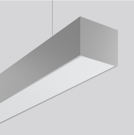
Luminaires suspendus 4051859973034 L 1691, B 110, H 88 suspension argent, mat (env. RAL 9006)
