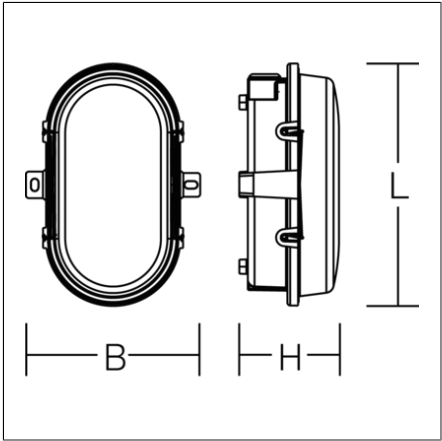
Ovale armaturen uit kunststof 4051859946779 L 171, B 123, H 70 Plafondmontage (opbouw), Wandmontage grijs
