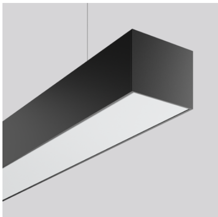
Pendant luminaires 4051859954088 L 1411, B 110, H 88
