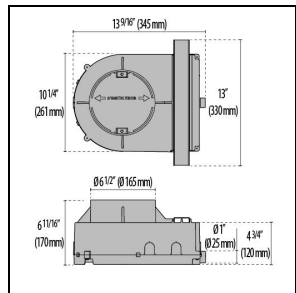
3111136 Inbouwdoos
