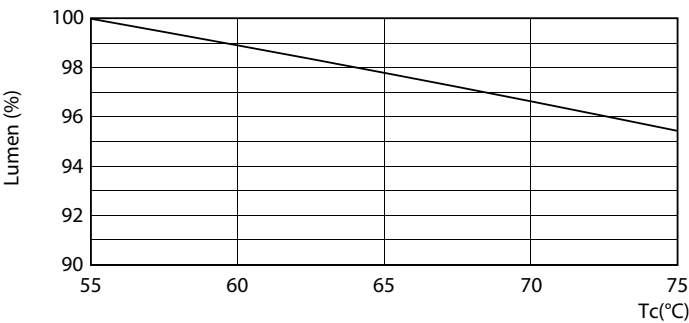
TLED_220-240V_G13-LumenVsTc
