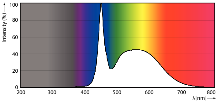
TLED_4ft_220-240V_15.5-36W2500lm_6500K_G13
