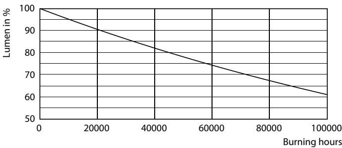
TLED_220-240V_G13
