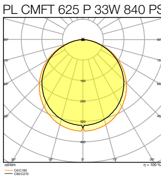
PL CMFT 625 P 33W 840 PS EM CONVERSION BOX
