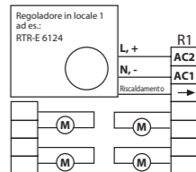
Valvole per locale 1 Válvulas para la sala 1
