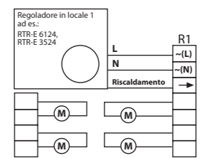
Valvole per locale 1
