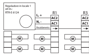
Valvole per locale 1 Valvole supplementari per locale 1
