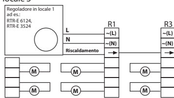
Valvole per locale 1 Valvole supplementari per locale 1
