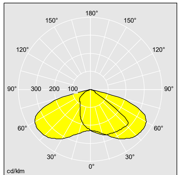
TL_UAS24L50NR740.ltd
